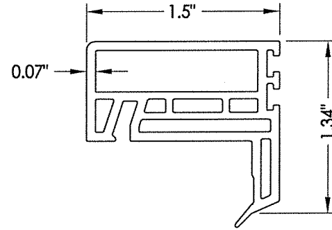
7 LOCK STILE
